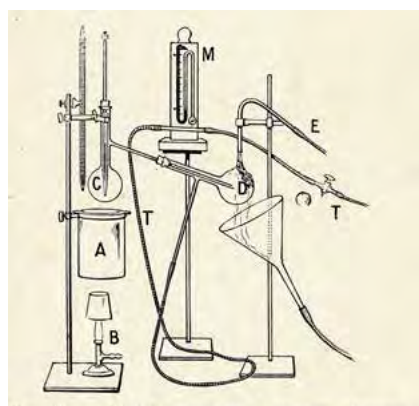
FIG. 20. — DISTILLATION SOUS PRESSION RÉDUITE.
