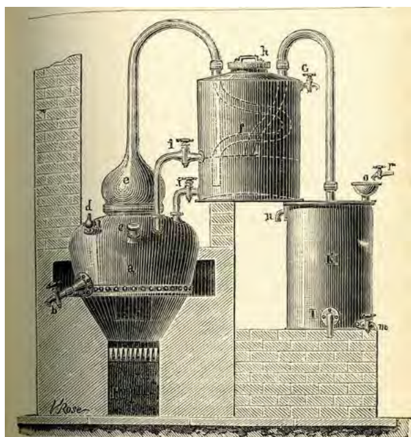
Fig. 9. — Brûleur à chauffe-vin installé dans un fourneau en maçonnerie. a. Chaudière en cuivre étamé. — b. Robinet de vidange. — c. Bouchon à vis pour l'emplissage. — d. Robinet d'air. — e. Chapiteau. — f. Chauffe-vin. — g. Robinet de jauge. — h. Tampon d'emplissage. — i. Sortie de l'eau-de-vie. — j. Robinet de vidange du chauffe-vin. — k. Réfrigérant. — l. Robinet de vidange du réfrigérant. — m. Trep-plein. — n. Entonnoir.
